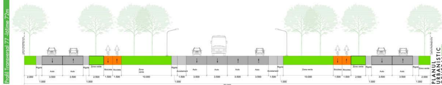
Sectiune conform Anexa 6 PUG Timisoara, Faza3, 2013, se propune profilul stradal transversal PTT77 pentru DN 69
